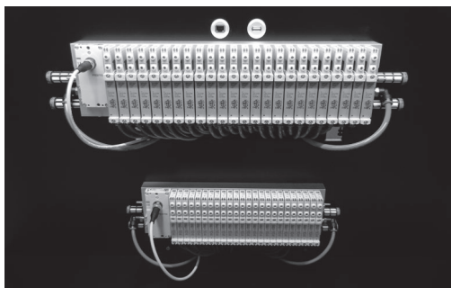
コンパクトでも大流量 - コストパフォーマンスの高い VTUG バルブターミナルがアクチュエータへ圧縮空気を供給
