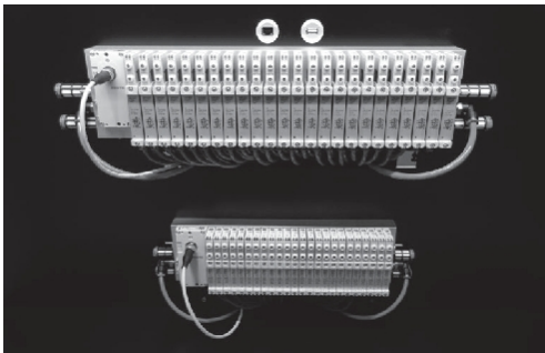
높은 유속의 컴팩트한 사이즈 - 비용 효율적인 밸브 터미널 VTUG는 액추에이터에 압축 공기를 공급합니다.
